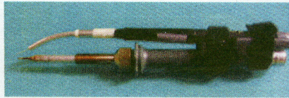
溶かしたはんだが出る事で片手で扱える「半手(ハンディ)こて」
